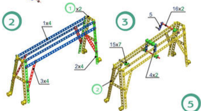
Мостовой кран
