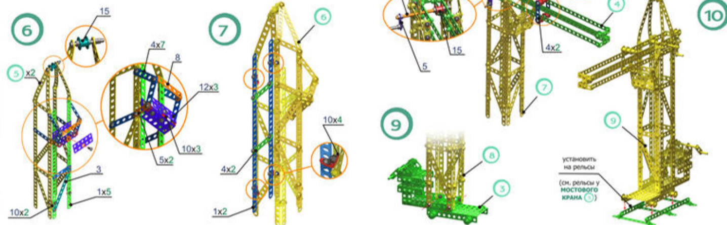
Башенный кран
